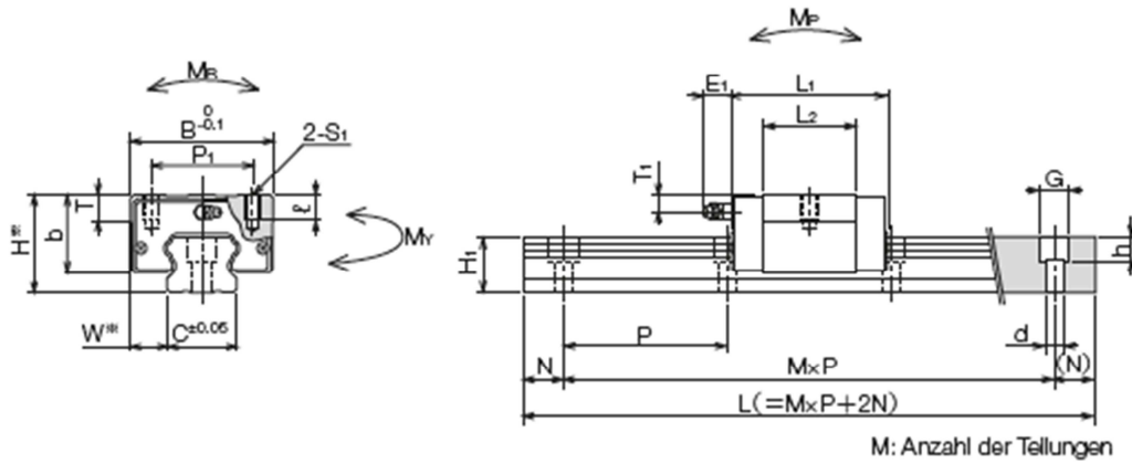
Laufwagen MGN-C / MGN-H
