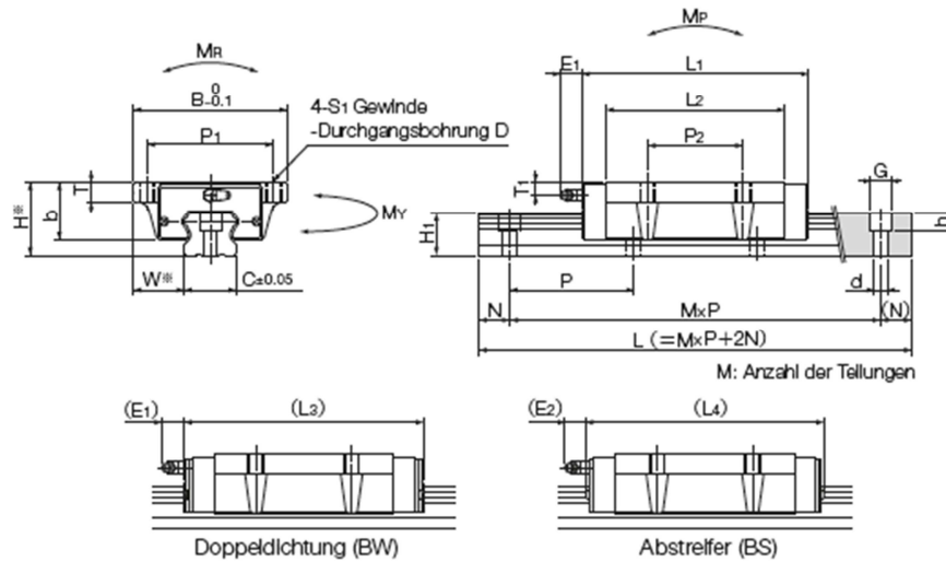
Laufwagen SGL-HYE
