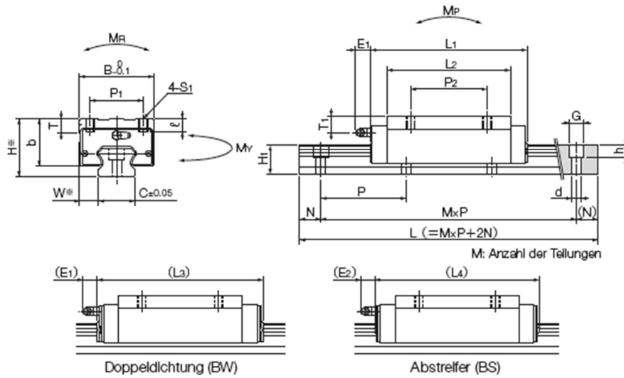
Laufwagen SGL-HTF
