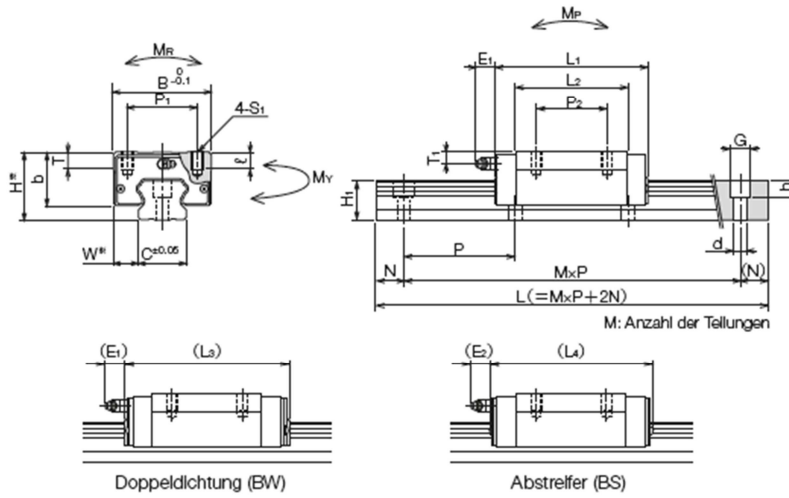
Laufwagen SGL-TF
