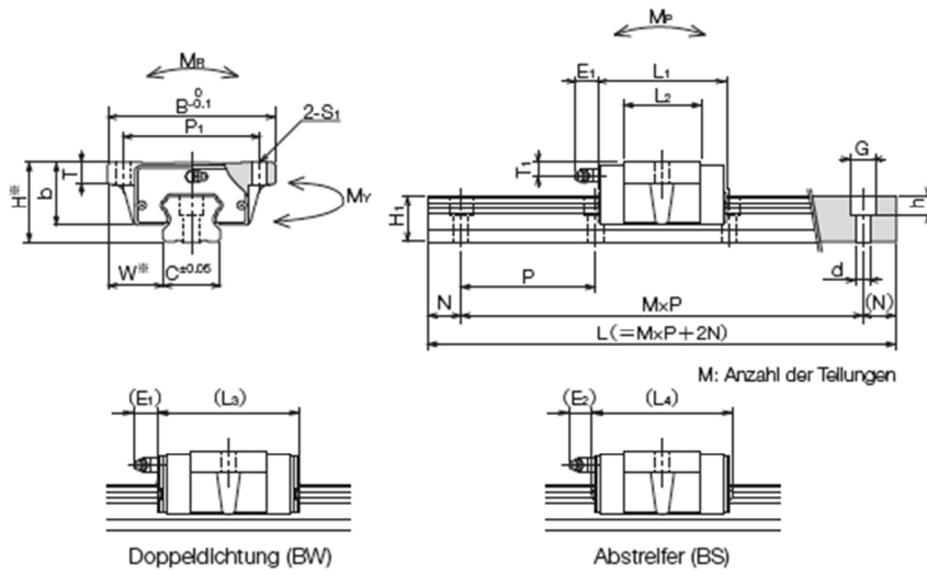
Laufwagen SGL-E
