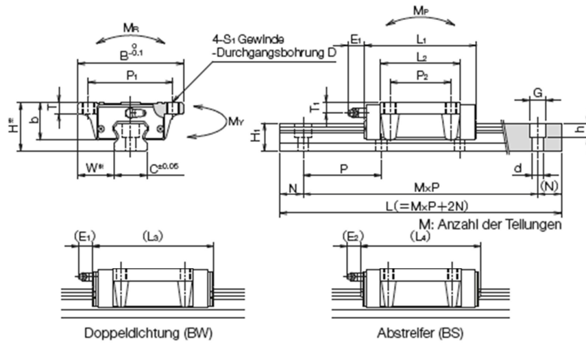
Laufwagen SGL-HTE
