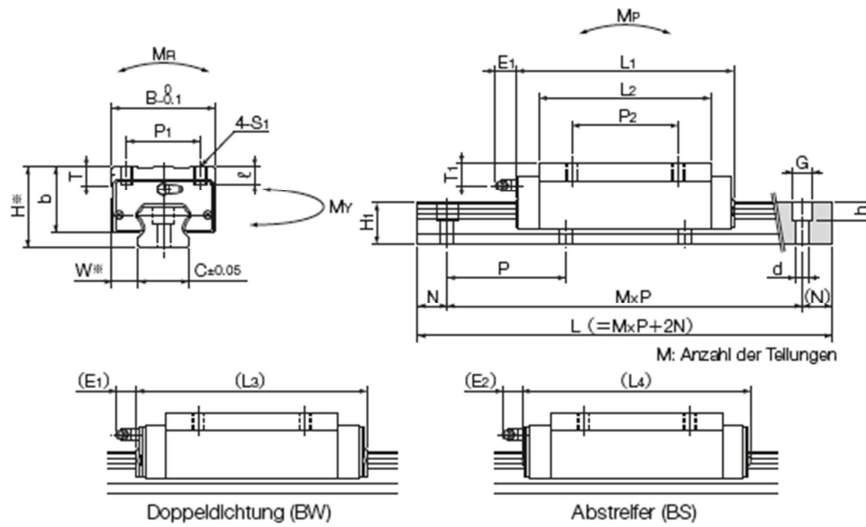
Laufwagen SGL-HYF
